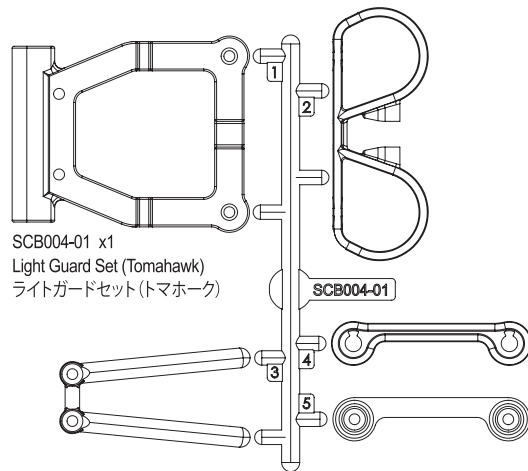
LA43 x3 5.8mm Ball End ボールエンド 5.8φ
